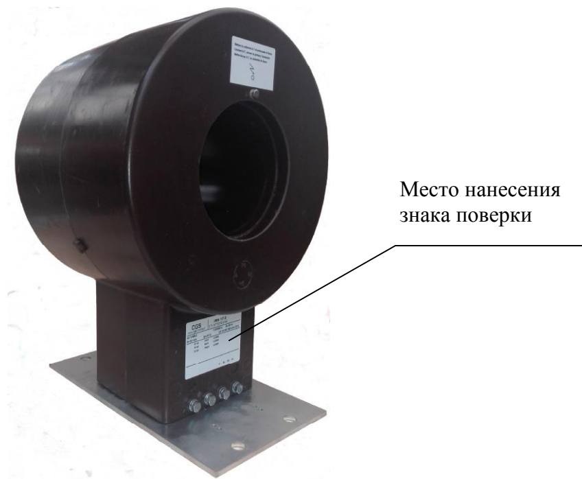
Рисунок 1 – Общий вид трансформаторов
