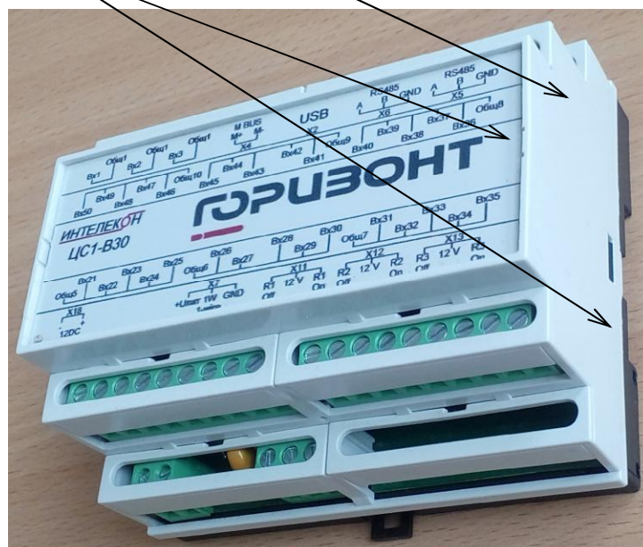
Рисунок 1 – Общий вид УСПД: а) ИНТЕЛЕКОН - ШД, б) ИНТЕЛЕКОН - ЦС1
