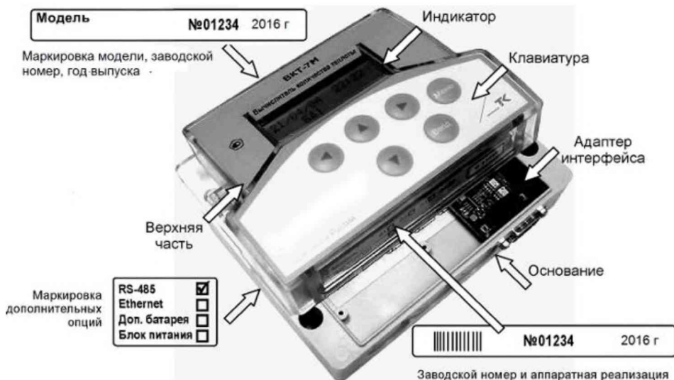
Рис. 3.1 – Внешний вид ВКТ-7М
