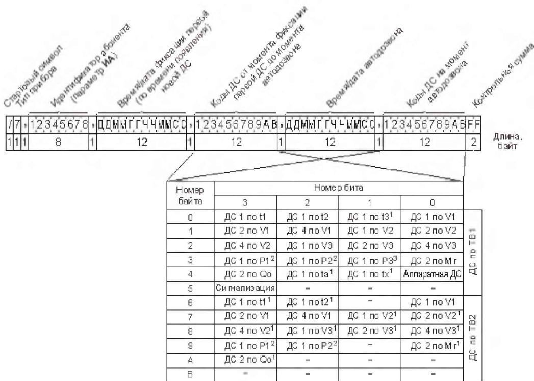
Рис. К.1 – Структура SMS сообщения
