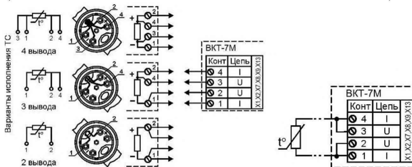
а) Подключение ТС по 4-проводной схеме
