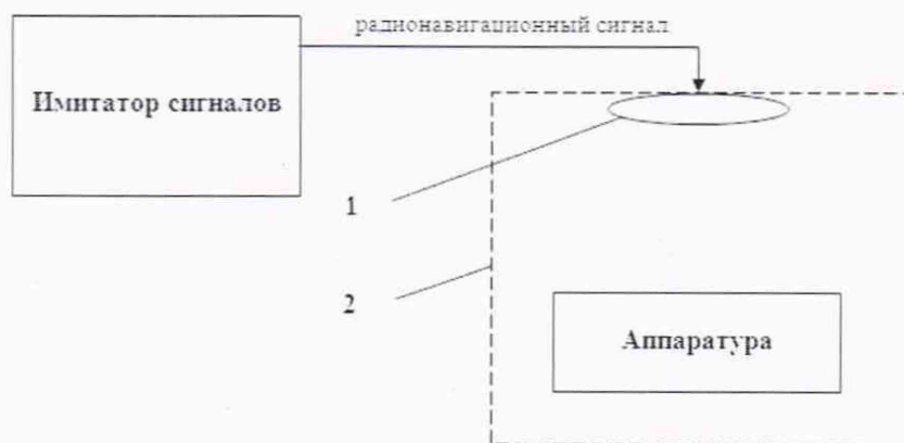
Рисунок 1 – Схема измерений
