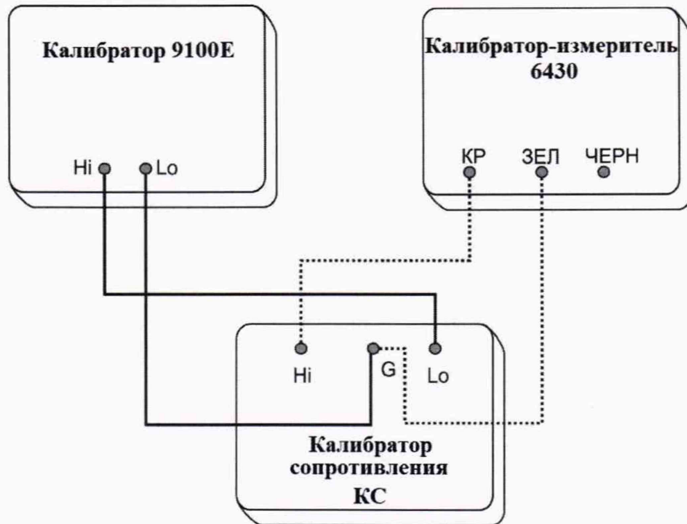
Рисунок 1 – Схема соединения оборудования
