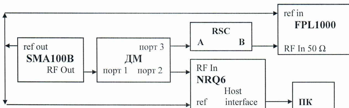
Рисунок 6 – Структурная схема соединения СИ для определения абсолютной погрешности измерений отношения мощностей в диапазоне измерений уровней мощностей
