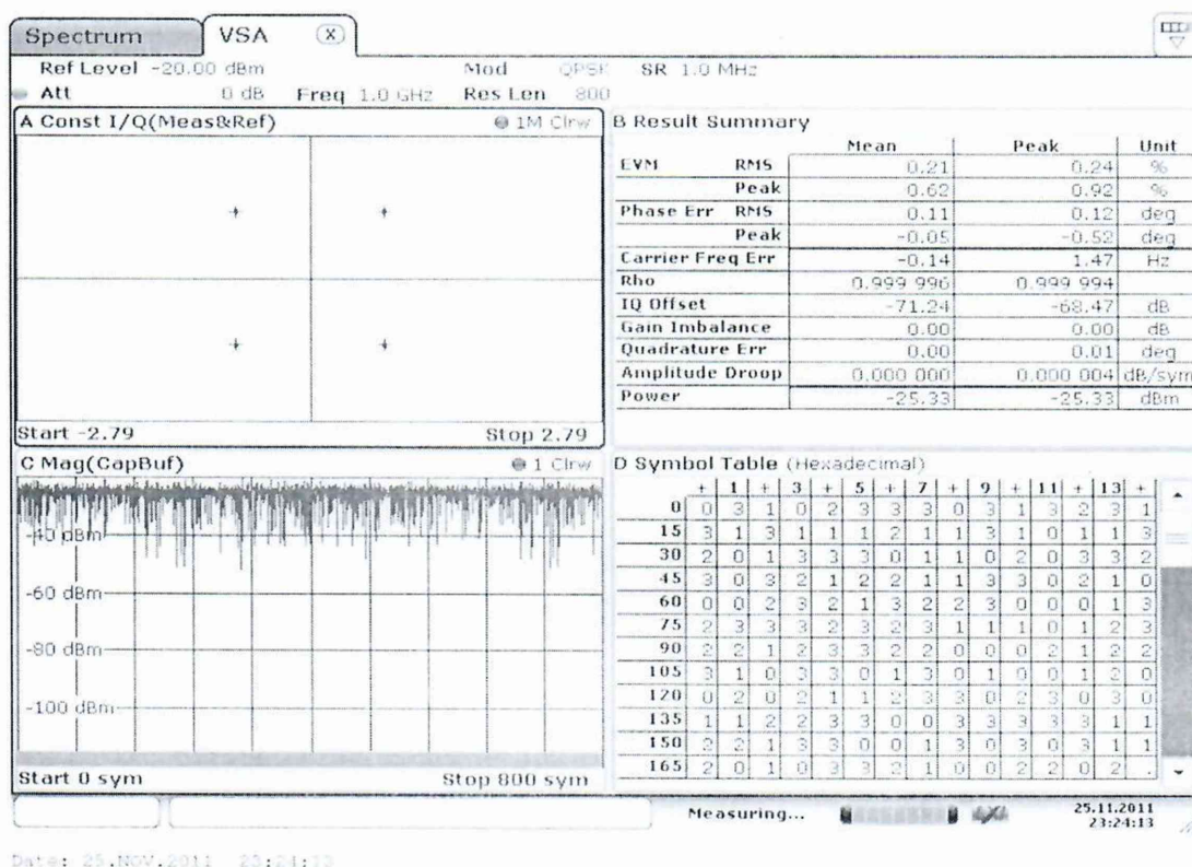
Рисунок 10 – меню анализатора в режиме измерений модуляции типа QPSK
