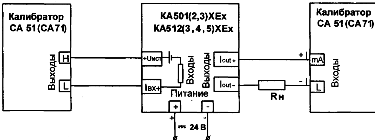
Рисунок 6.5.2 – Подключение барьеров мод. KA5011Ex, KA5012Ex, KA5013Ex, KA512XEx, KA513XEx, KA514XEx, KA515XEx для проверки преобразования входных унифицированных сигналов постоянного тока (входной пассивный сигнал) в диапазоне от 4 до 20 мА в выходной унифицированный сигнал постоянного тока от 4 до 20 мА
