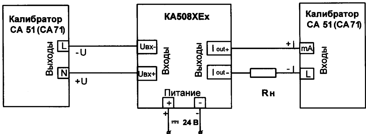
Рисунок 6.9.1– Подключение барьера КА508ХЕх для поверки преобразования сигналов напряжения в диапазоне от минус 5 до 0 В, выходной сигнал - ток от 4 до 20 мА
