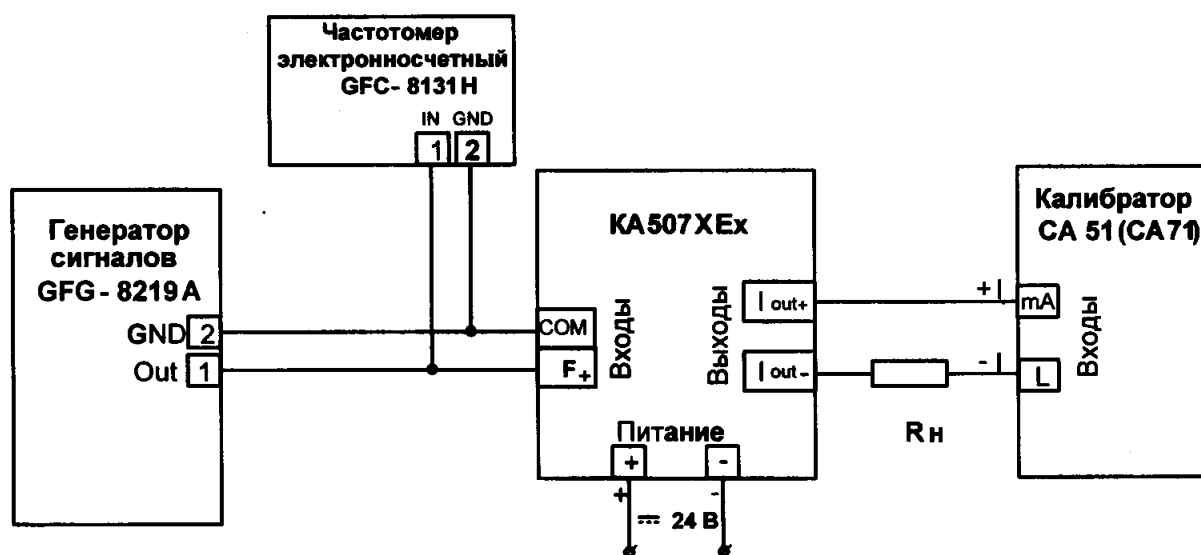
Рисунок 6.8.1. – Схема подключения барьера КА507ХЕх для поверки преобразования частоты периодического импульсного сигнала в выходной унифицированный сигнал постоянного тока в диапазоне от 4 до 20 мА
