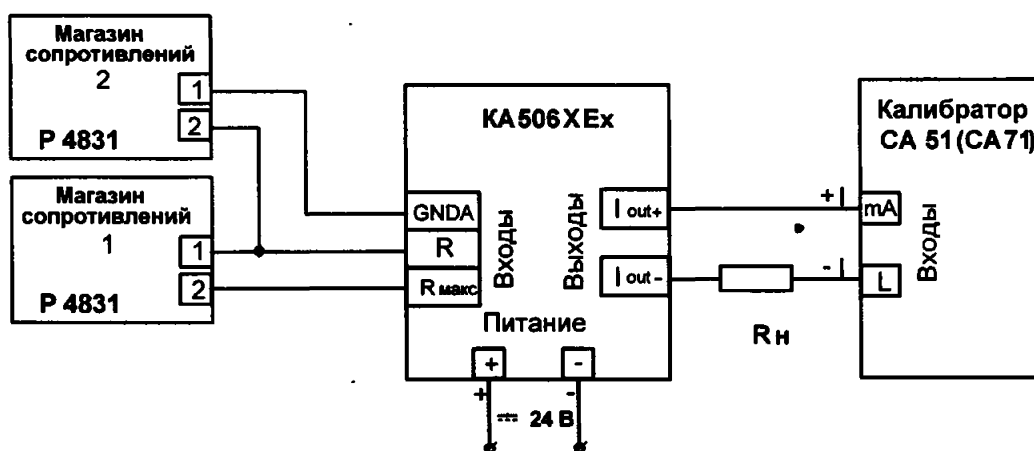
Рисунок 6.7.1– Подключение барьера КА506ХЕх для поверки преобразования положения потенциометрических датчиков в диапазоне от 0 до 100 % в унифицированный сигнал постоянного тока от 4 до 20 мА
