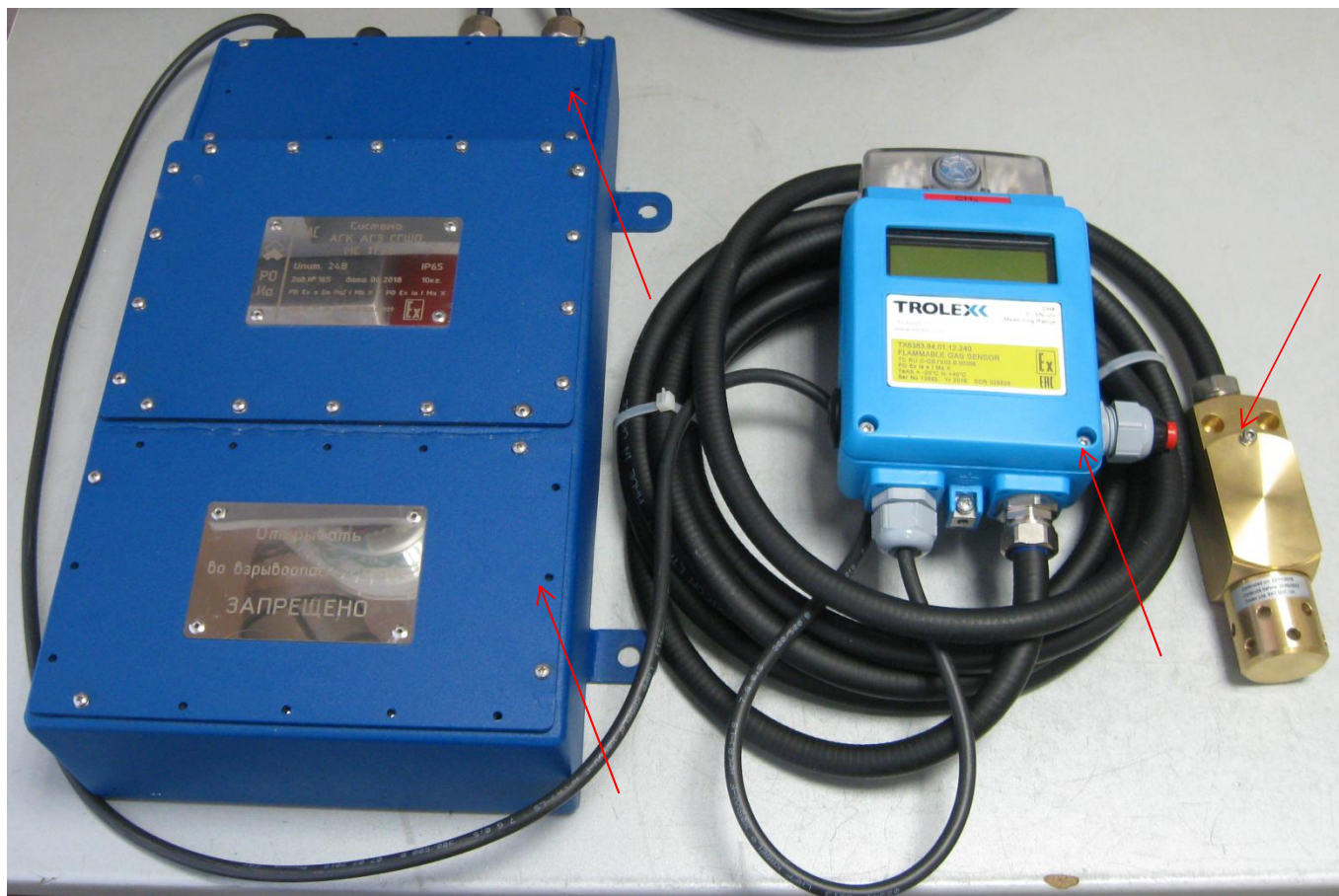
б) MS 11.26-01 с датчиком метана TX6383.84
