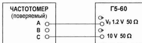
Рисунок 8.1 - Схема подключения приборов при измерении интервалов времени
