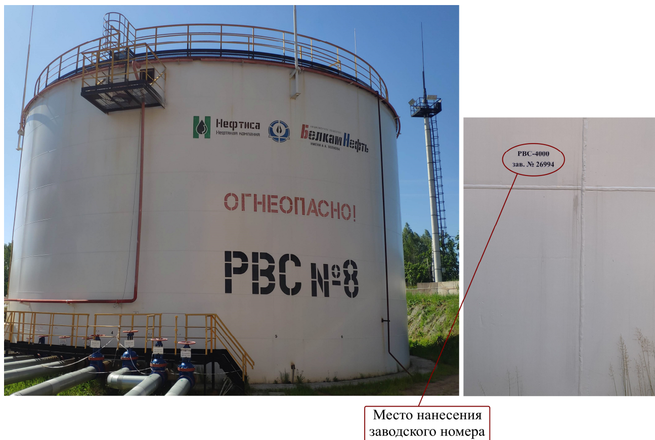
Рисунок 1 – Общий вид резервуара РВС-4000 №26994 с указанием места нанесения заводского номера
