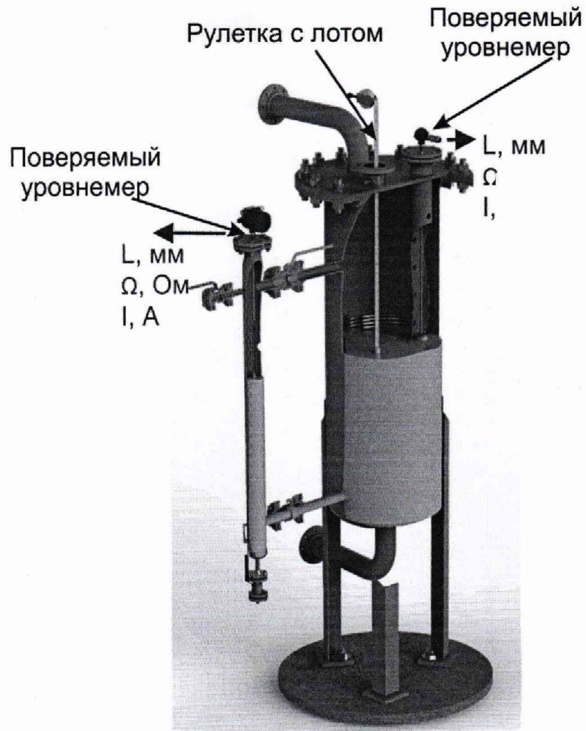
Рисунок 2 – Проверка датчика уровня без демонтажа с помощью эталонной рулетки с лотом
