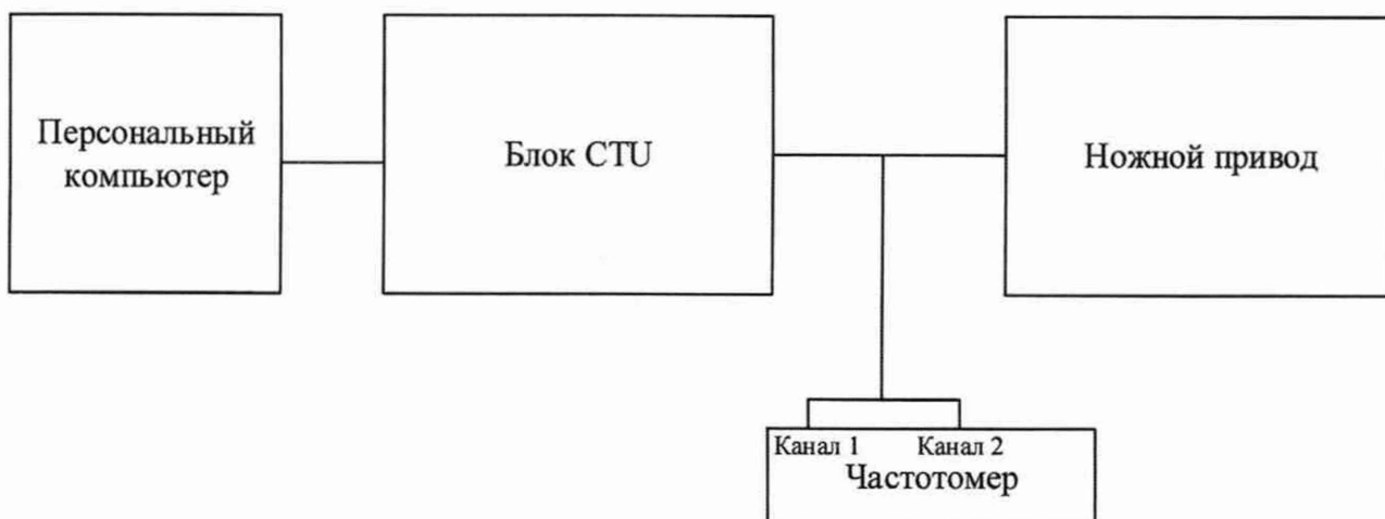
Рисунок 1 – Схема подключения при определении абсолютной погрешности измерений интервала времени
