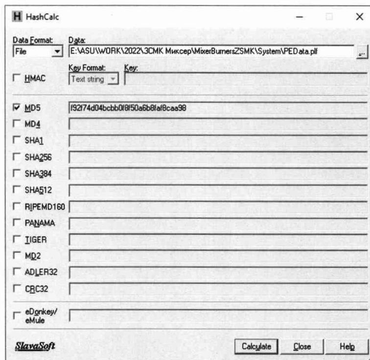
Рисунок 1 – Расчет контрольной суммы MD5 файла конфигурации проекта
