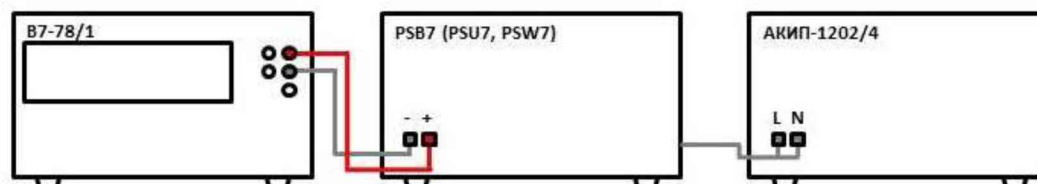
Рисунок 1 – Схема подключения приборов при определении абсолютной погрешности воспроизведения напряжения постоянного тока
