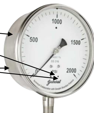
Рисунок 2 – Места нанесения знака утверждения типа и заводского номера
