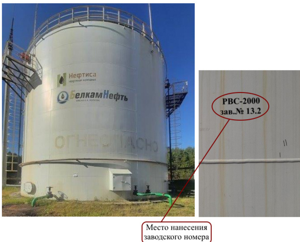
Рисунок 1 – Общий вид резервуара PBC-2000 №13.2 с указанием места нанесения заводского номера
