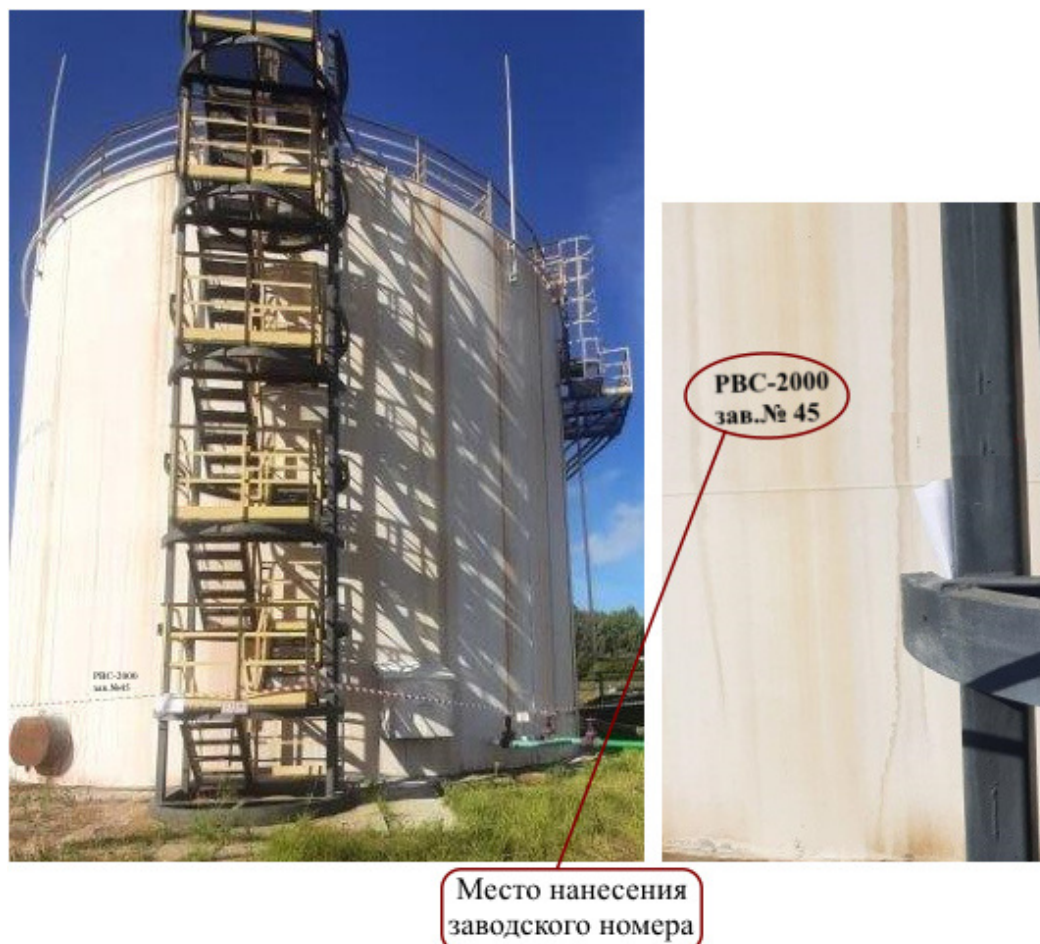
Рисунок 3 – Общий вид резервуара РВС-2000 №45 с указанием места нанесения заводского номера
