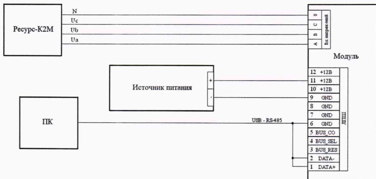
Рисунок Б.1– Схема подключения измерительных цепей
