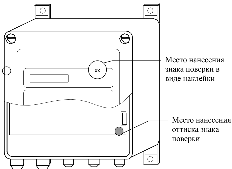
Рисунок 3 – Схема пломбирования теплосчетчика ТЭМ–104 поверителем
