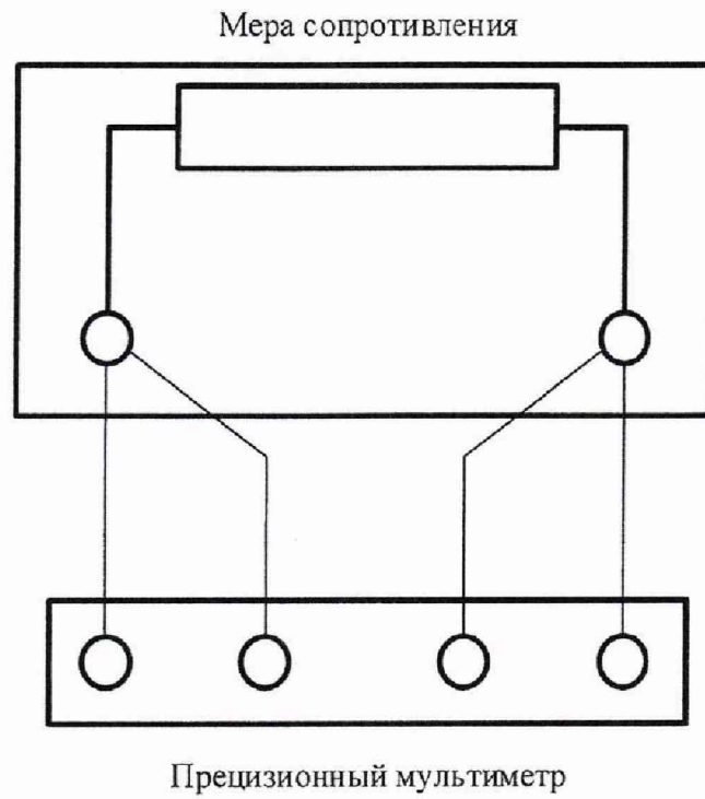
Рисунок А.7- Схема подключения прецизионного мультиметра
