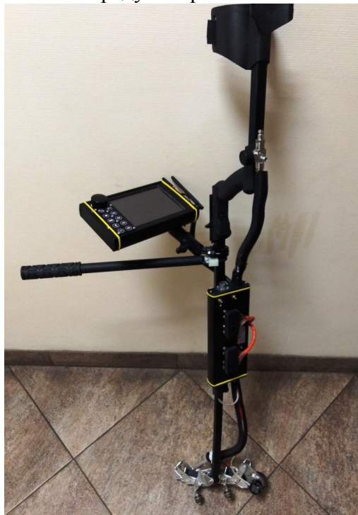
Рисунок 1 – Общий вид дефектоскопов ультразвуковых однопиточных «СОМ»
