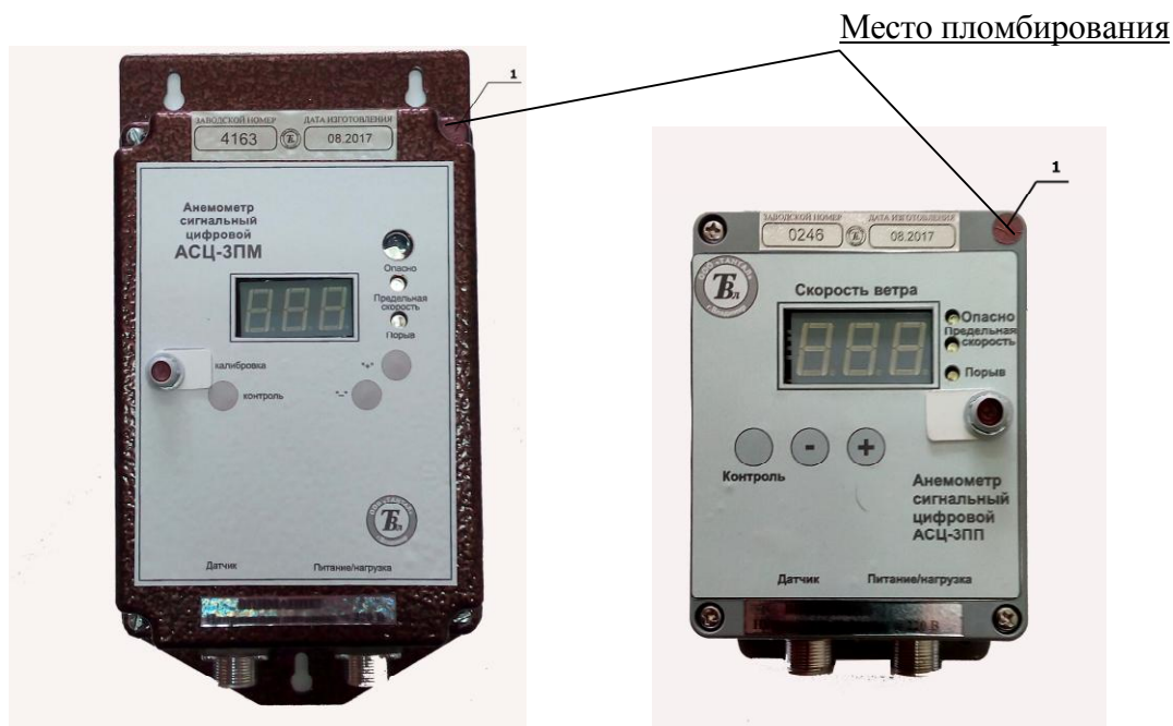
Рисунок 3 - Место пломбирования
