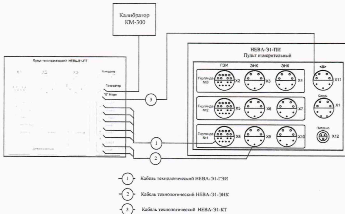
Рисунок 4 – Схема для определения метрологических характеристик измерений разности электрических потенциалов измерительных каналов
