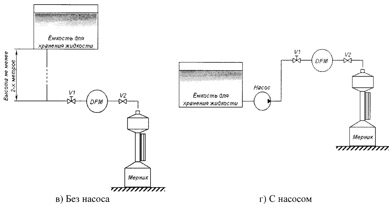
Рисунок Б.2 – Схемы поверки счетчика объемным методом
