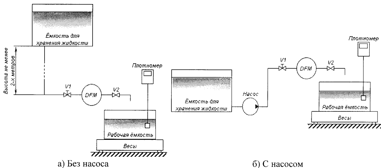
Рисунок Б.1 – Схемы поверки счетчика массовым методом
