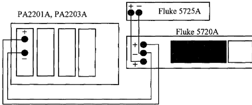
Рисунок 1 – Схема подключения при поверки постоянного и переменного напряжения
