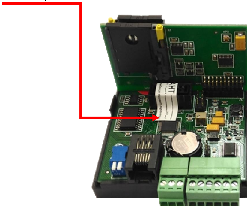
Рисунок 6 - Место пломбировки модуля М-320И
