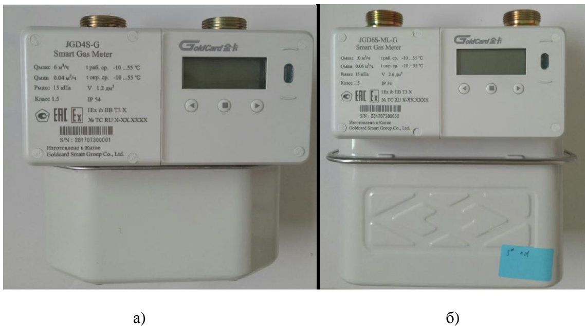
Рисунок 1 - Общий вид счетчиков и схема нанесения знака поверки и пломбы завода-изготовителя
