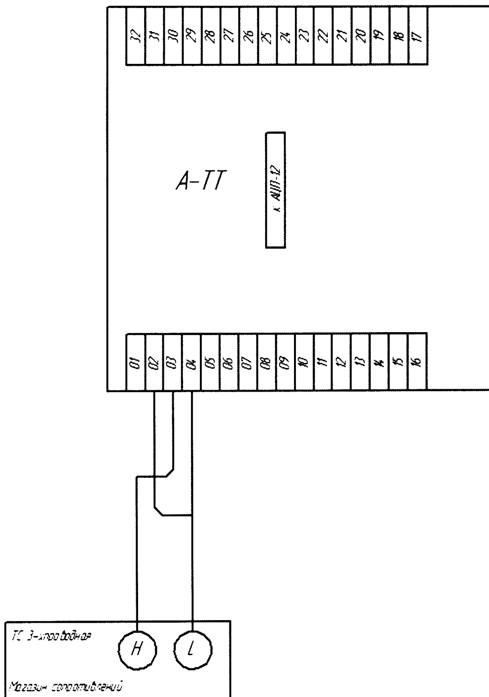
Рисунок Гб. Сигналы имитации термопреобразователей сопротивления (трехпроводная схема)
