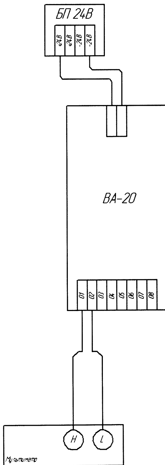
Рисунок Г11. Унифицированный токовый сигнал
