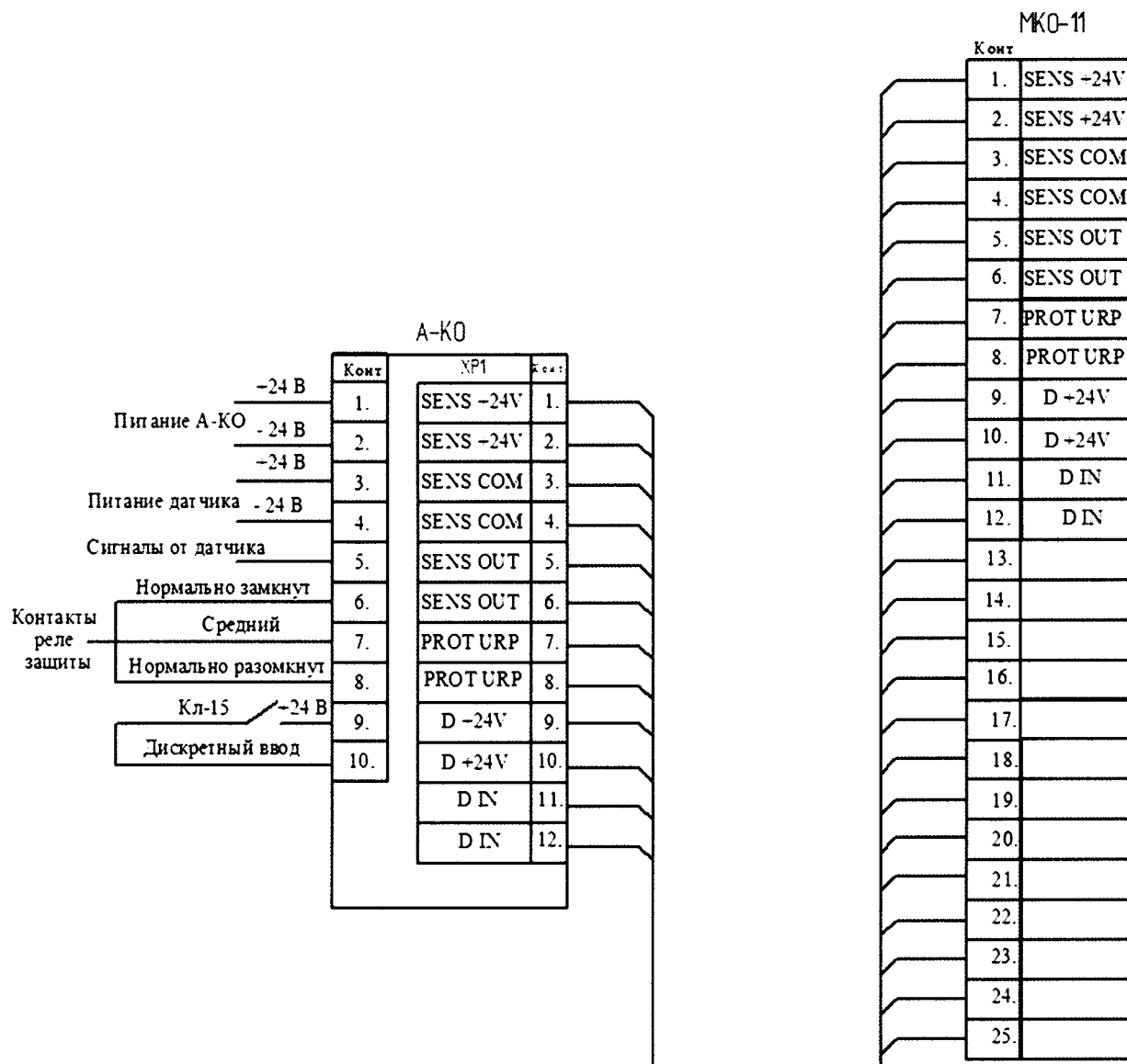
Рисунок В14. Сигнал от датчика частоты
