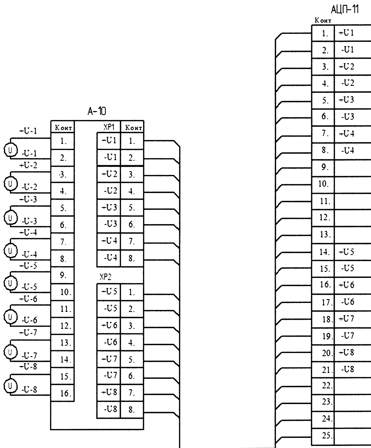
Рисунок В3. Напряжение постоянного тока высокого уровня
