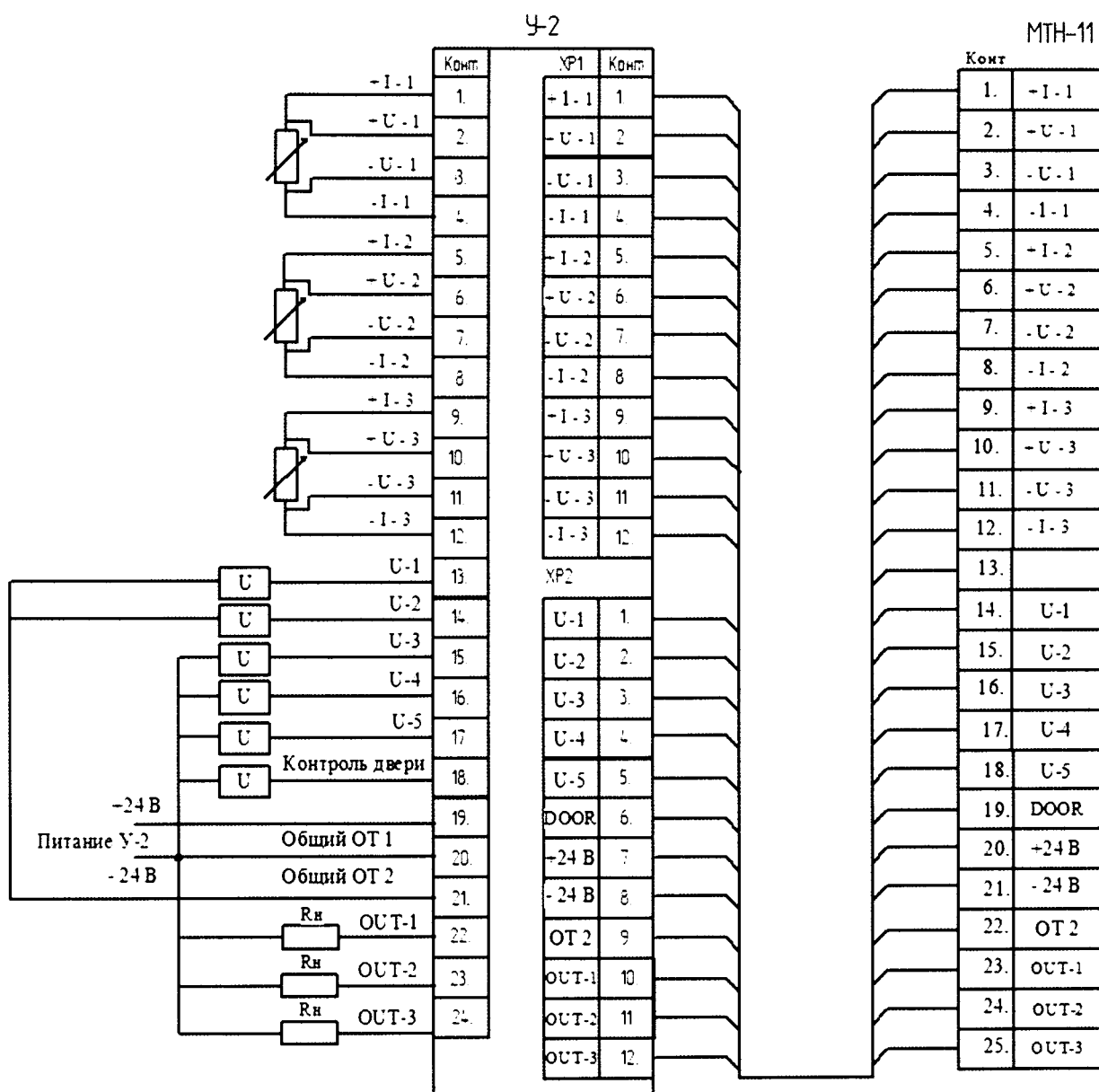
Рисунок В12. Три канала измерения температуры холодного слая (термопреобразователи сопротивления по ГОСТ6651-2009: Pt-100 \alpha=0,00385 с четырёхпроводной схемой подключения)
