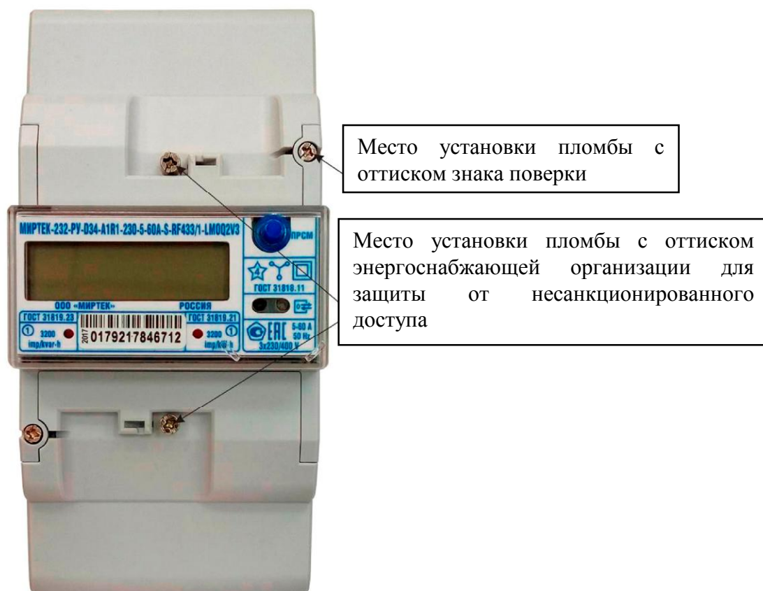
Рисунок 6 - Общий вид счетчика и схема пломбировки от несанкционированного доступа в корпусе типа D34
