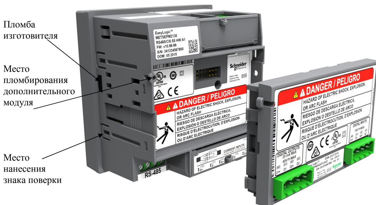
Рисунок 3 - Места опломбирования счетчиков серии PM2000 и дополнительного модуля
