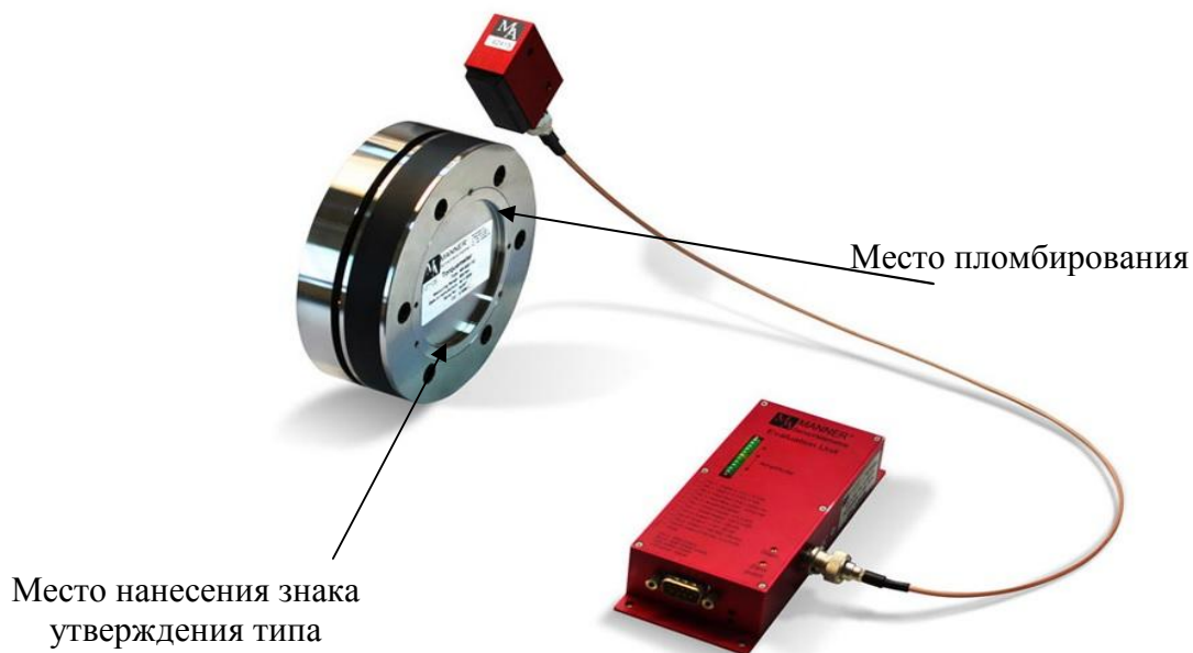
Рисунок 1 - Внешний вид измерителя крутящего момента силы MW
