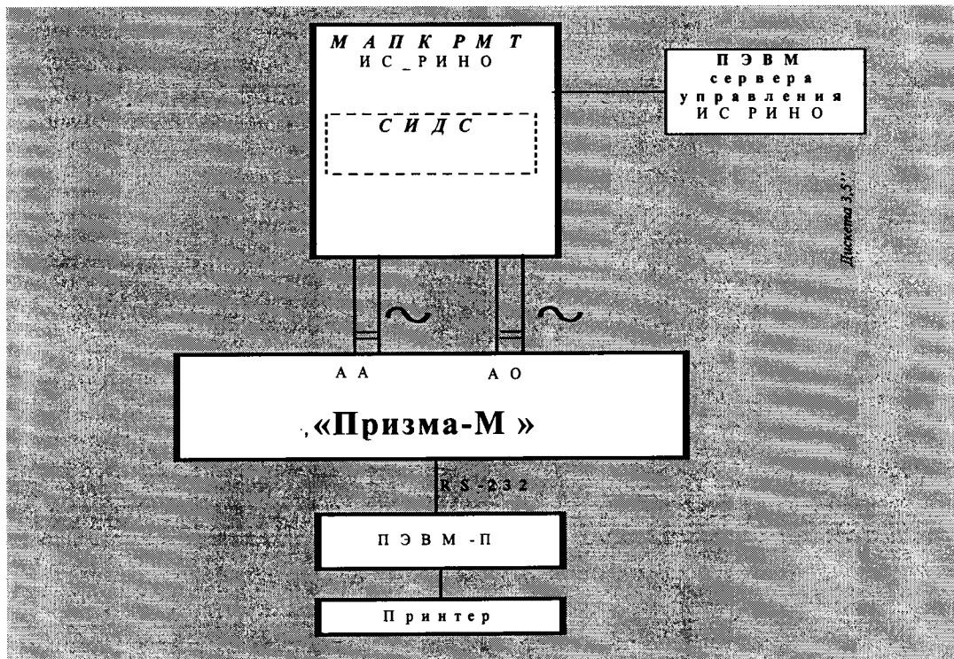
Рисунок 1. Схема поверки СИДС ИС РИНО
