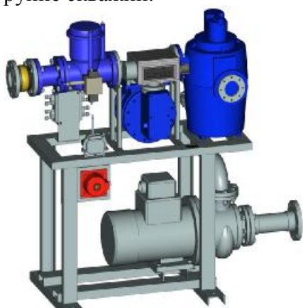
Исполнение со счетчиком жидкости
