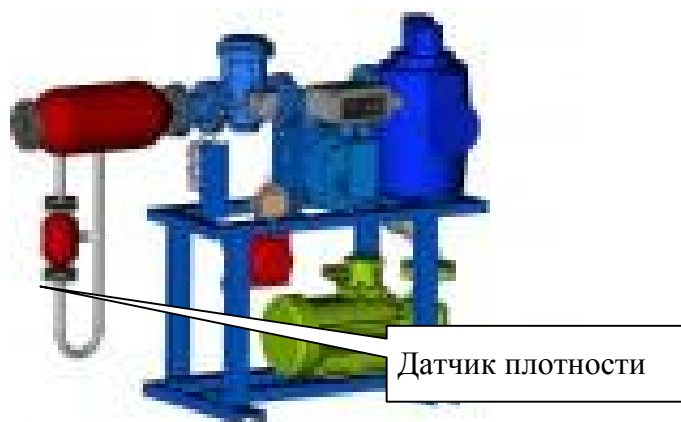
Исполнение со счетчиком и плотномером
