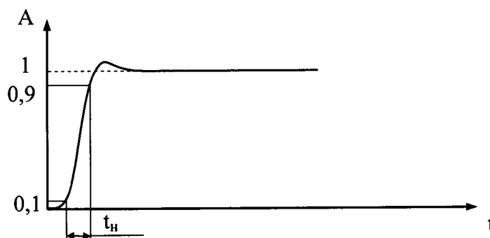
Рисунок 5 – Изображение испытательного импульса при измерении времени нарастания переходной характеристики тизм.
