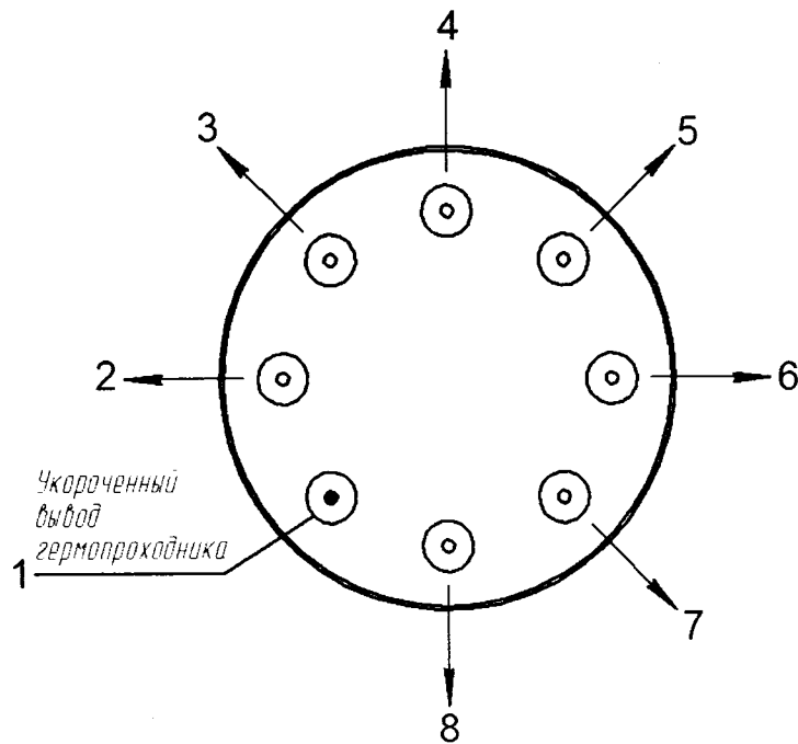
Рисунок 2 – выводы преобразователя
