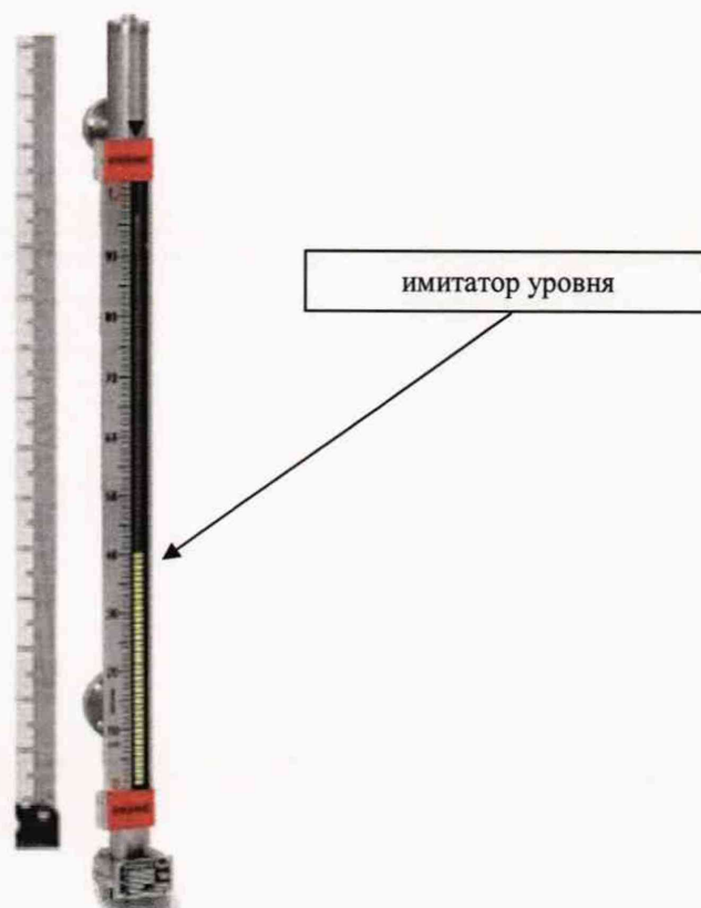
Рисунок Б.1 - Поверка уровнемера с имитацией изменения уровня
