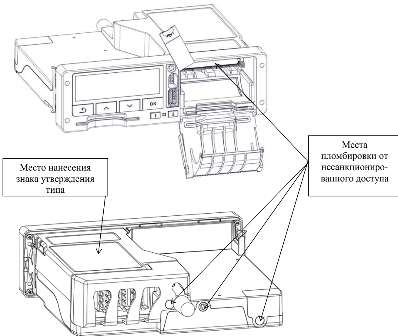
Рисунок 2 – Схема пломбировки от несанкционированного доступа и место нанесения знака об утверждении типа
