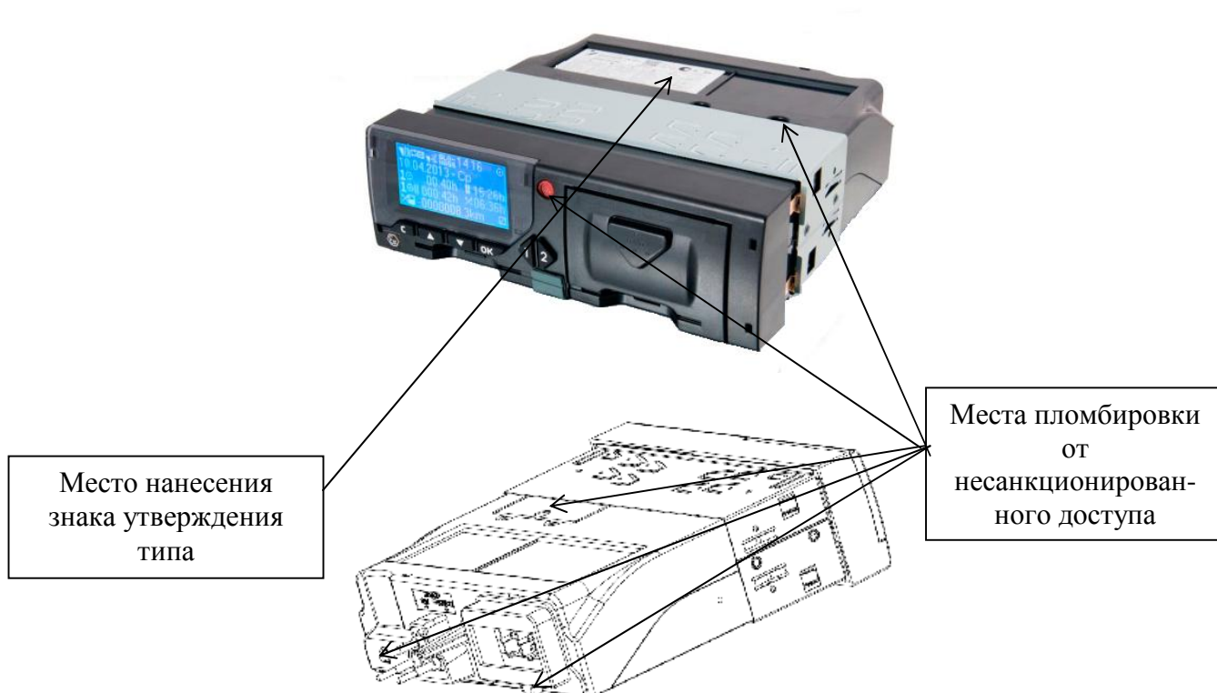
Рисунок 2 – Схема пломбировки от несанкционированного доступа и место нанесения знака об утверждении типа
