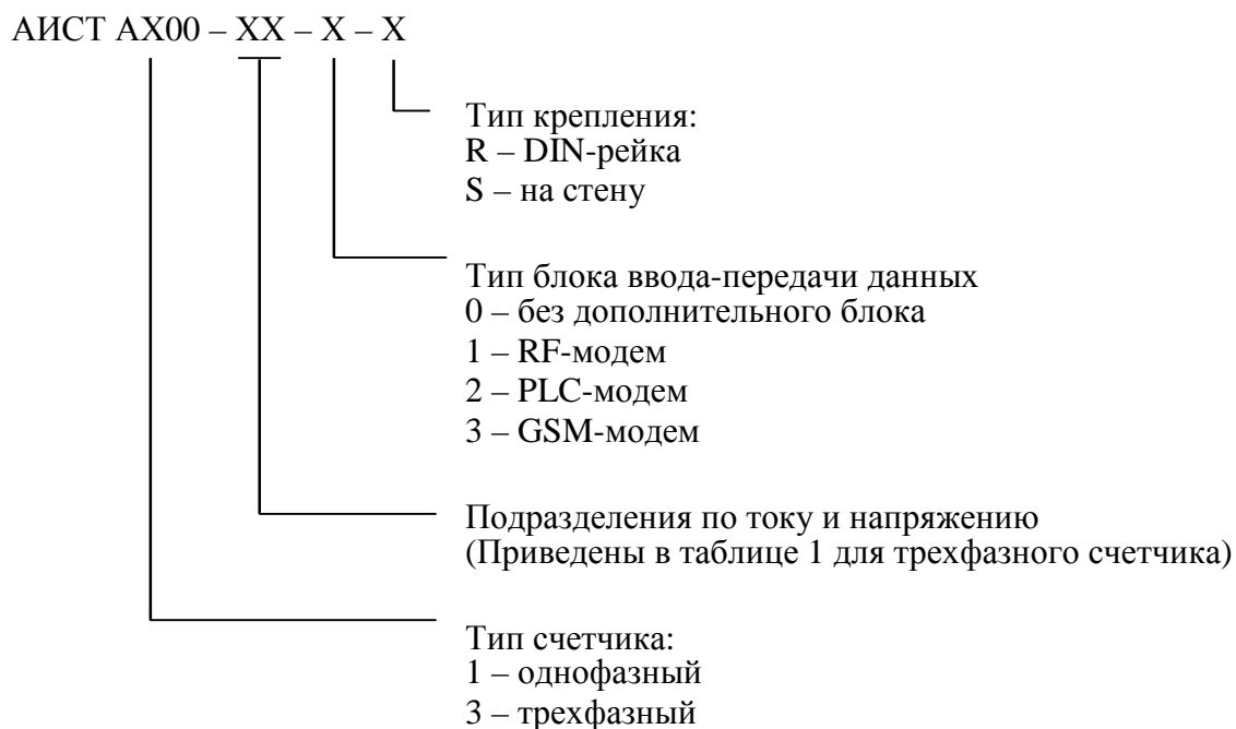
Рисунок 1. Структура условного обозначения счетчика
