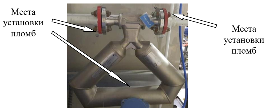
Рисунок 2 – Схема пломбировки от несанкционированного доступа счетчика-расходомера массового Micro Motion модели CMF100 с измерительным преобразователем серии 2700**
