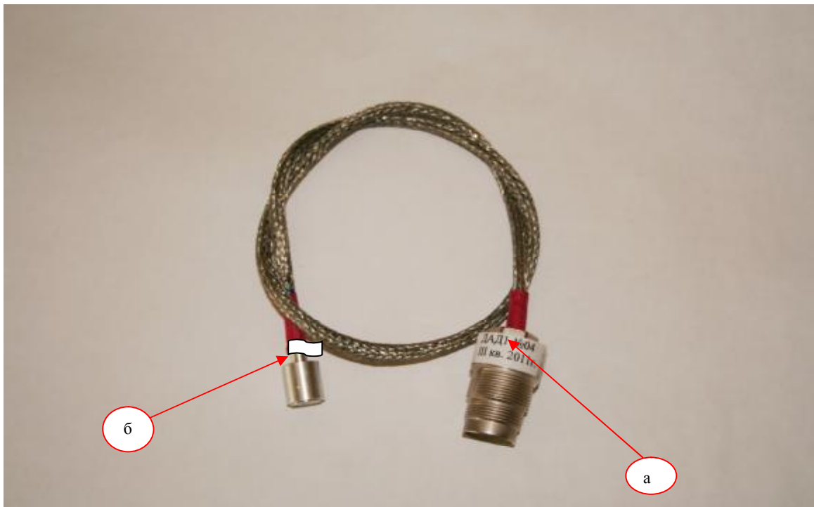
Рисунок 2 – Место нанесения наклейки (а) и пломбировки (б) детектора ДАД1
