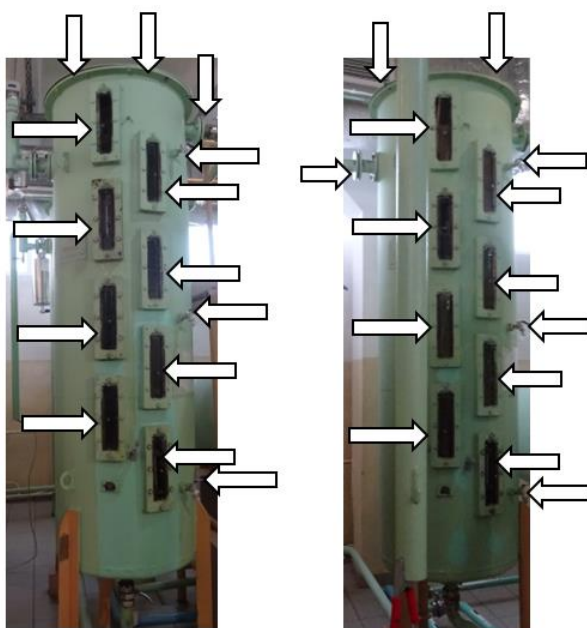
Рисунок 2 – Схема пломбировки мерников К7-ВМА, зав.№№ 462, 463 от несанкционированного доступа, обозначение места нанесения знака поверки.
