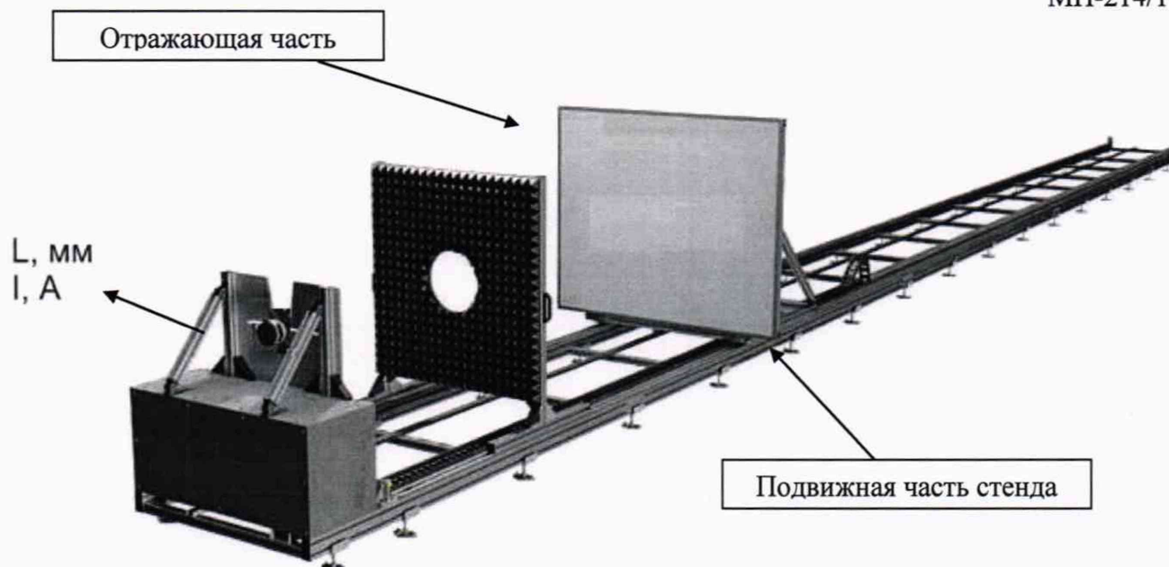
Рисунок 2 - Проверка уровнемера на поверочной установке с имитацией изменения уровня
