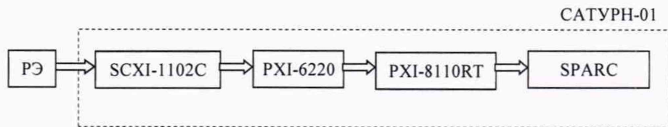
Рисунок 9 – Схема поверки ИК силы постоянного тока
