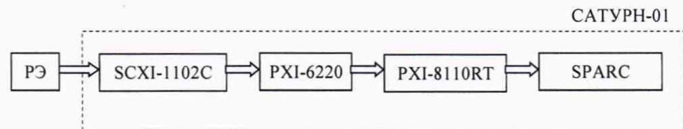
Рисунок 5 – Схема поверки ИК параметров вибрации
