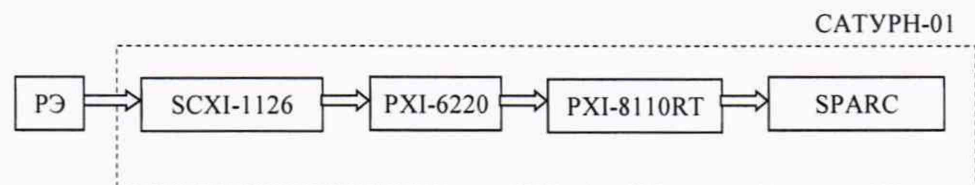
Рисунок 4 – Схема поверки ИК частоты вращения роторов
