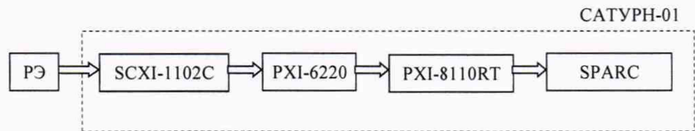
Рисунок 2 – Схема поверки ИК давления поэлементным способом
