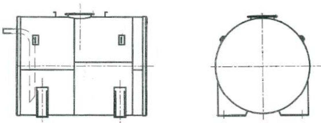
Рисунок 1 – Общий вид эскиза резервуара РГС-4
