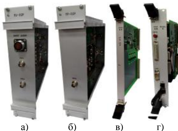
а) – Субблок ПУ-02Р; б) – Субблок ПР-02Р; в) – Модуль ВЧС; г) – Модуль ФП8
