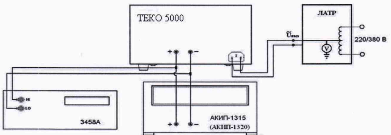
Рисунок 1 – Структурная схема соединения приборов.
