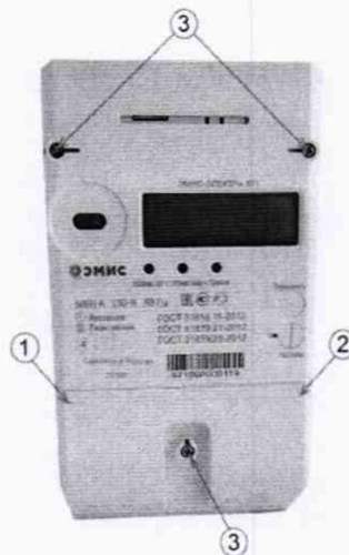
Рисунок 2 – Схема пломбировки счётчиков ЭМИС-ЭЛЕКТРА 971 исполнения «Х»
