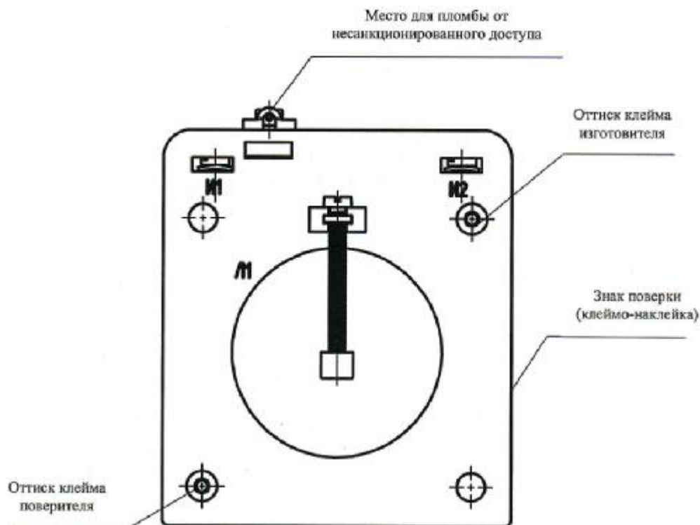
Рисунок 2 - Схема пломбировки от несанкционированного доступа и обозначение места нанесения знака поверки
