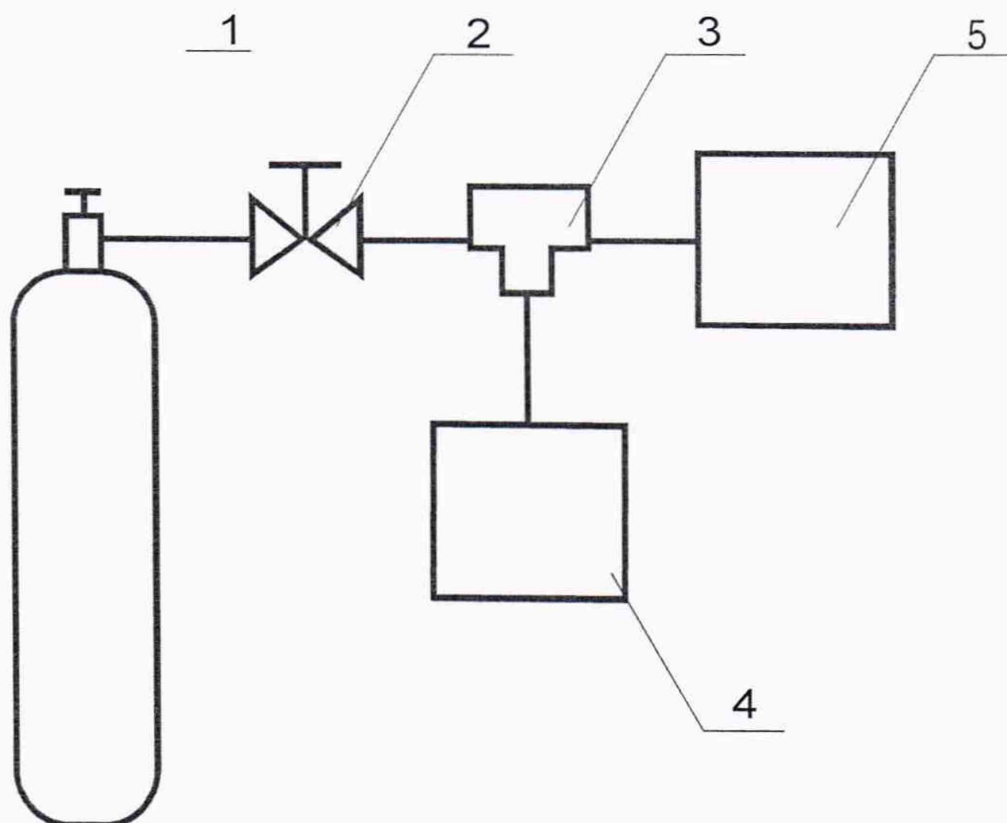
Схема подачи газовоздушной смеси
