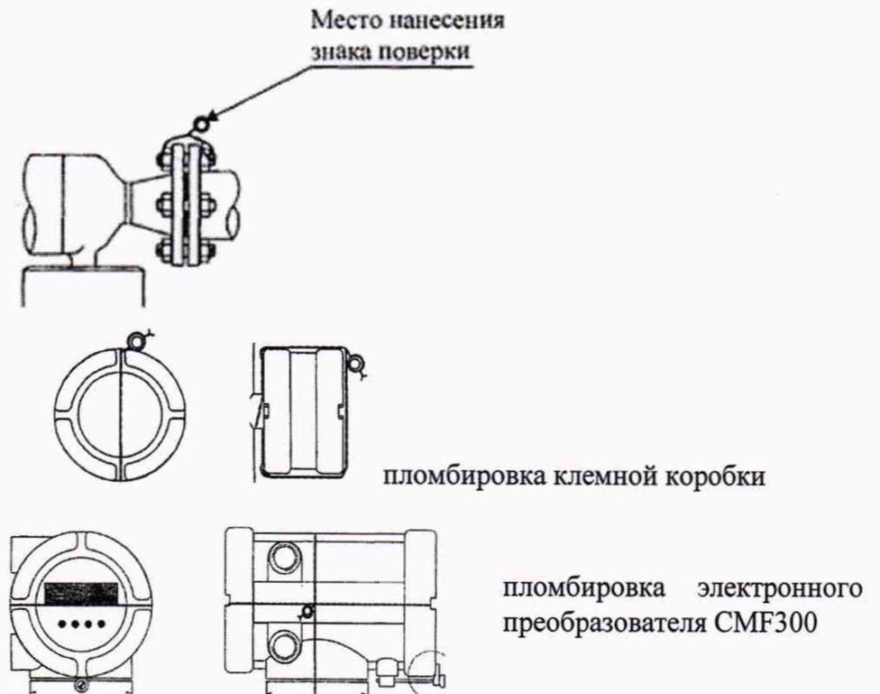
Рисунок Б.1 - Схема пломбировки клемной коробки, электронного преобразователя и фланцев счетчика-расходомера массового СМF300
